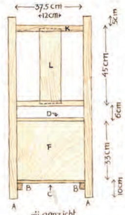
zij-aanzicht
