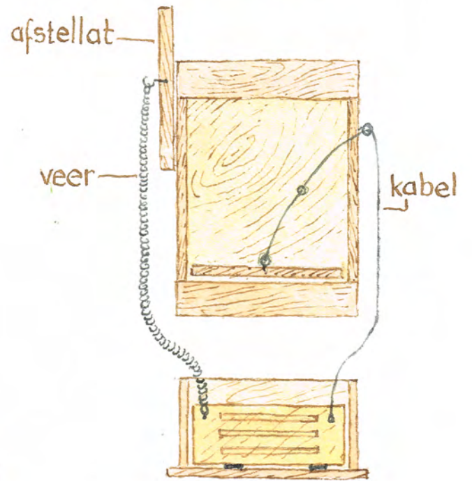
vooraanzicht
