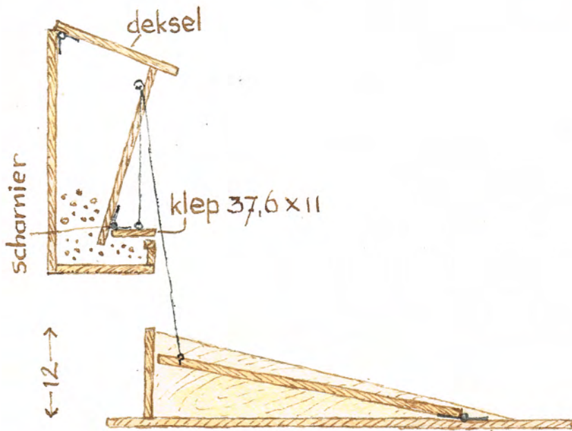
doorsnede voerbak
